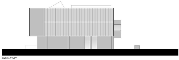
ANSICHT OST
