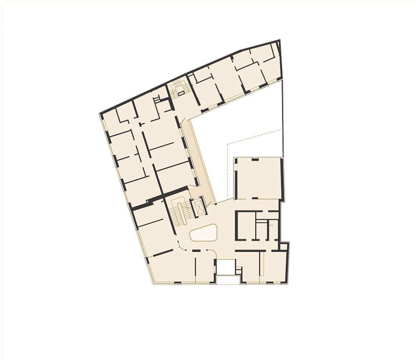
Grundriss OG1
