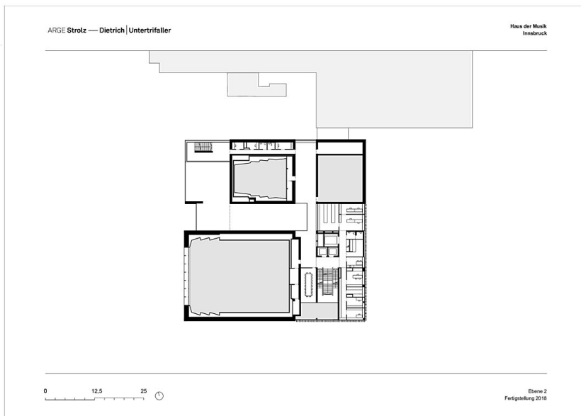
Grundriss E2
