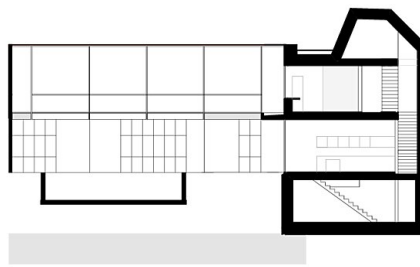
QUERSCHNITT
