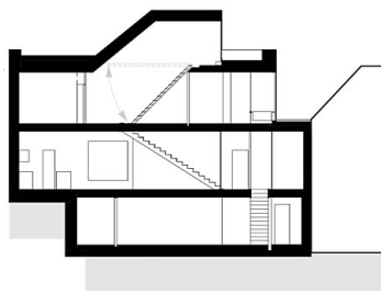
LÄNGSSCHNITT
