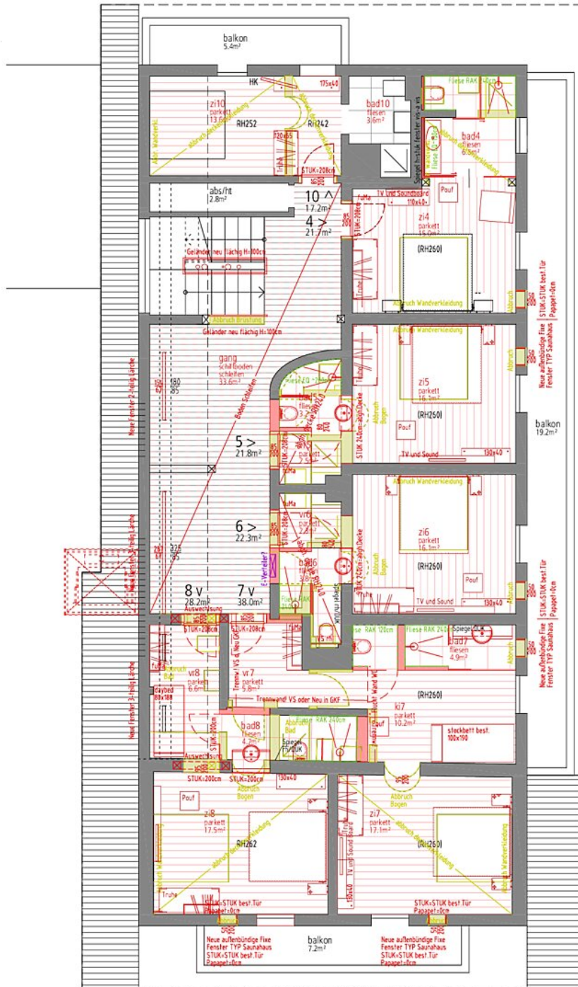
Grundriss OG2
