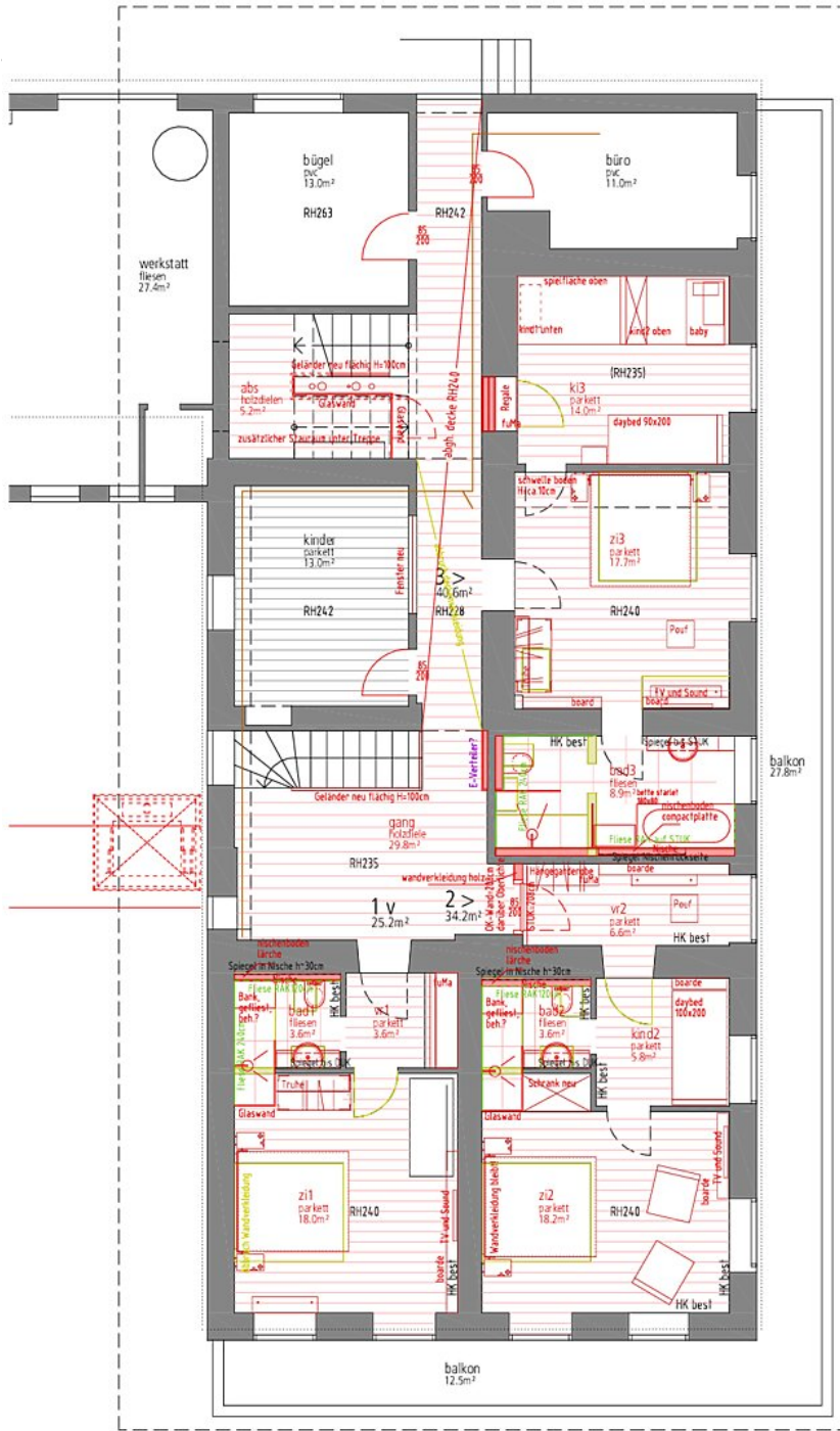
Grundriss OG1
