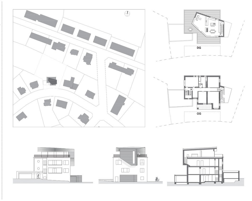
Lageplan, Grundrisse, Schnitt & Ansichten
