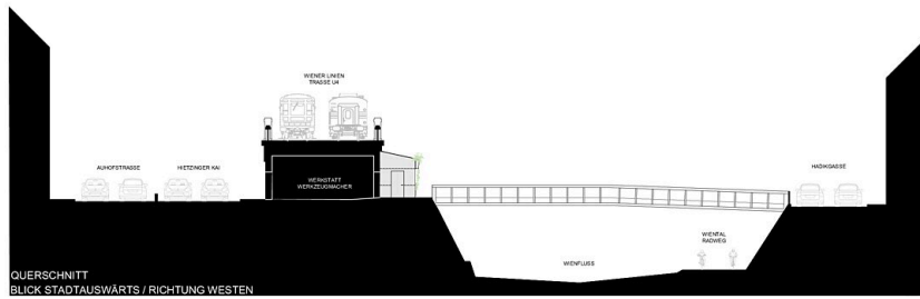
QUERSCHNITT BLICK STADTAUSWÄRTS / RICHTUNG WESTEN
