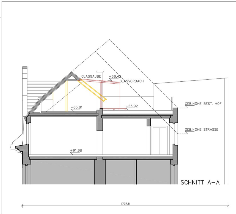
Schnitt AA
