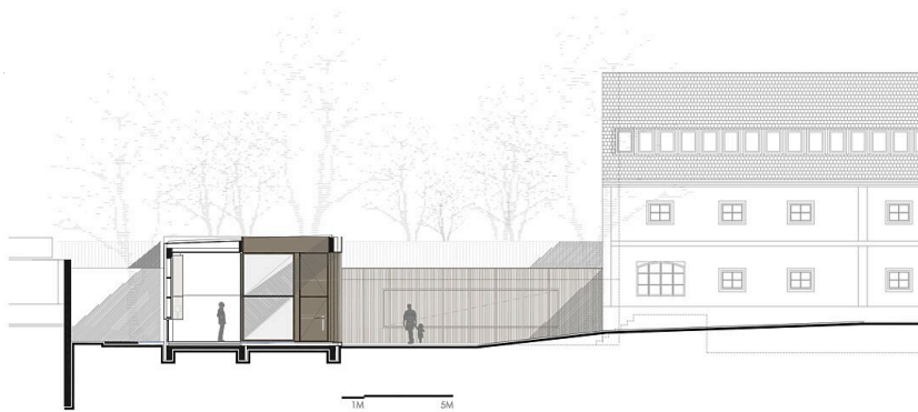
Schnitt B2
