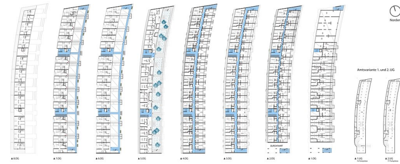
Grundrisse Riegel
