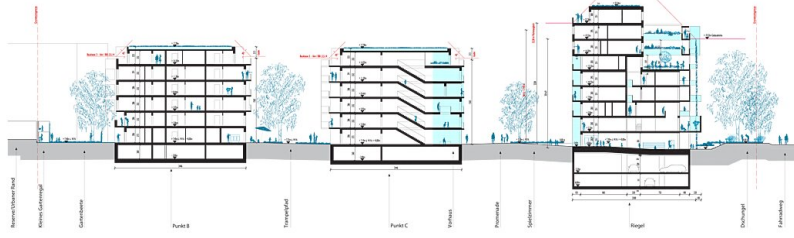
Schnitt
