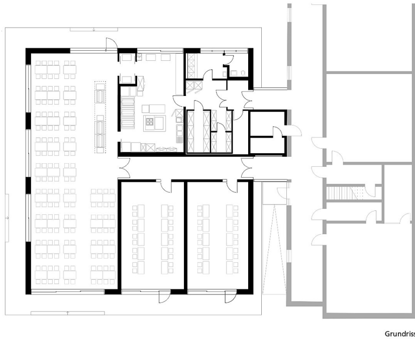
Grundriss
