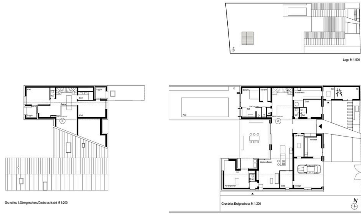
EFH SUA GRUNDRISSSE M 1:200
