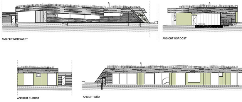
ANSICHTEN / 1:200
