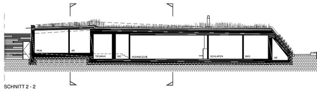
SCHNITT 2-2
