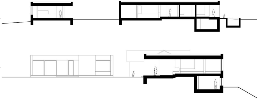
Doppelhaus Trausner Längsschnitt
