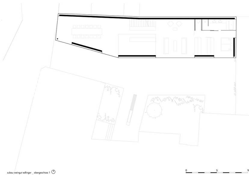
zubau weingut edlinger _ obergeschoss 1
