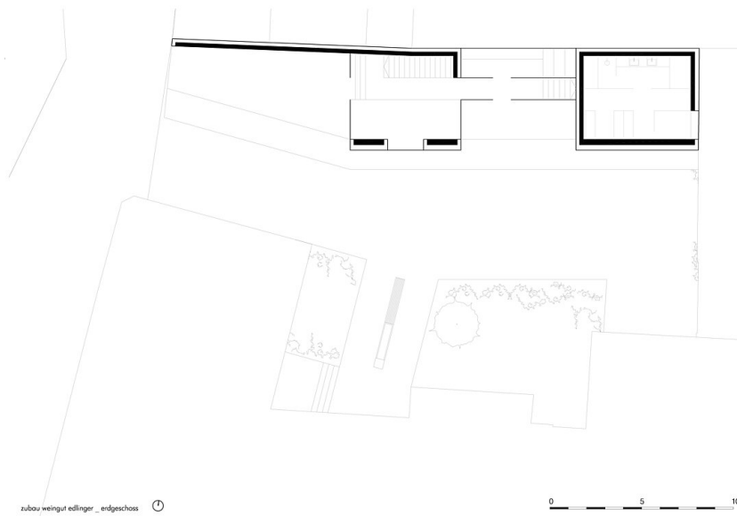
zubau weingut edlinger _ edgeschoss
