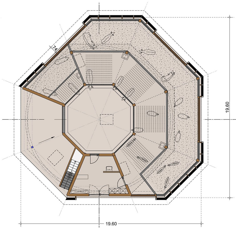
Grundriss EG
