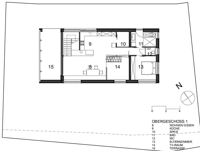
Grundriss OG 1
