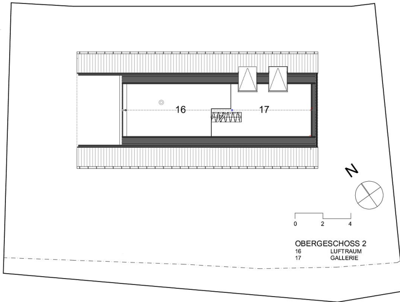
Grundriss OG 2
