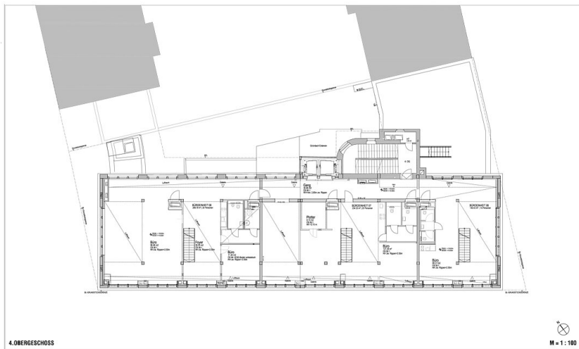
Grundriss OG4
