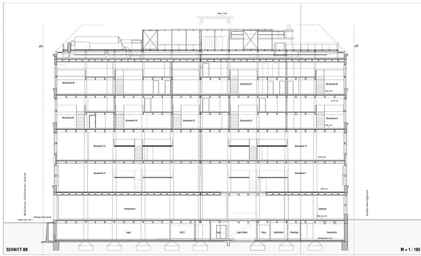
Schnitt B-B
