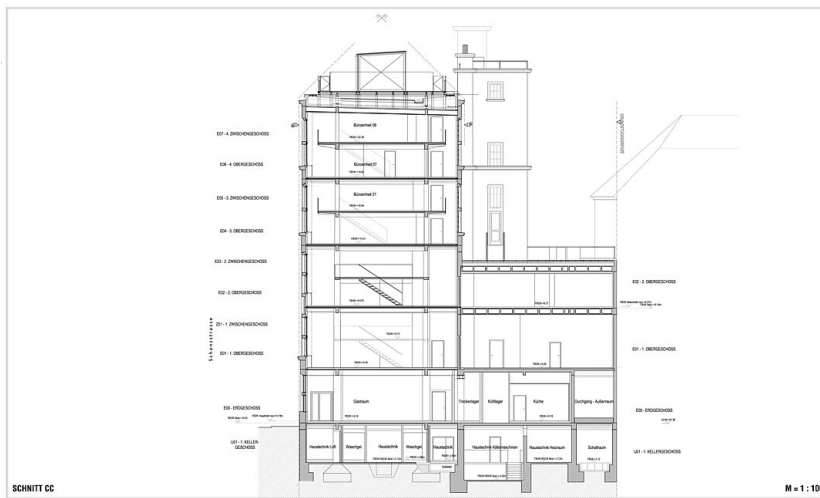
Schnitt C-C
