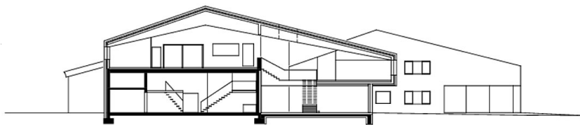
Querschnitt 1
