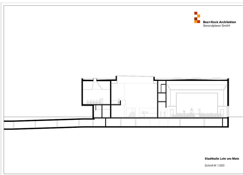
Schnitt 2
