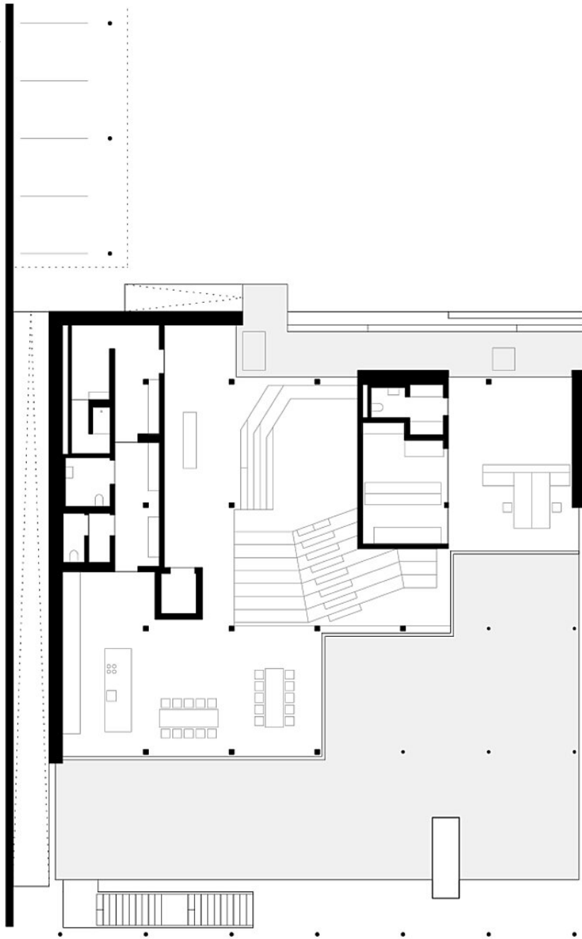
Grundriss OG
