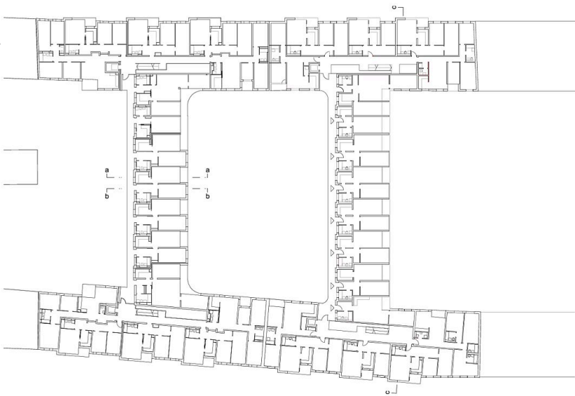
Grundriss RG
