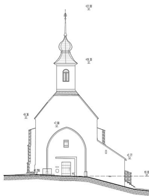
ANSICHT WEST
