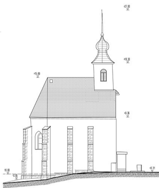
ANSICHT NORD
