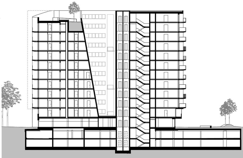
Längsschnitt
