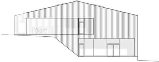
Ansicht Nord
