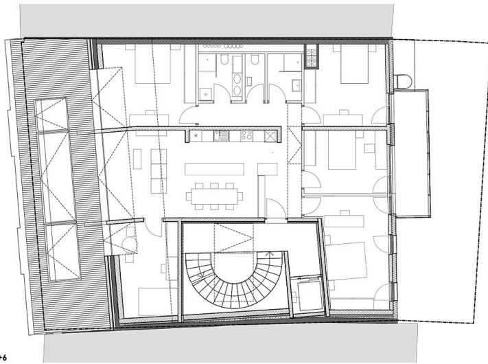
Grundriss OG6
