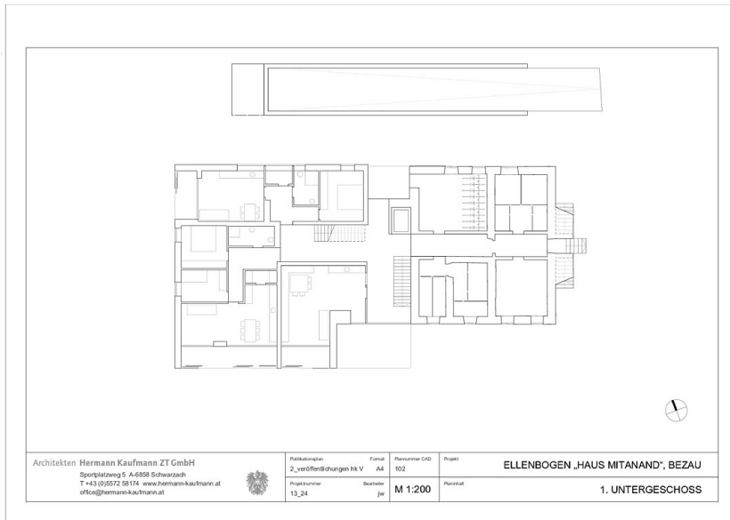
Grundriss UG1
