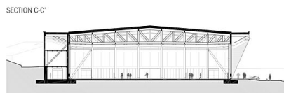
Schnitte, Ansichten
