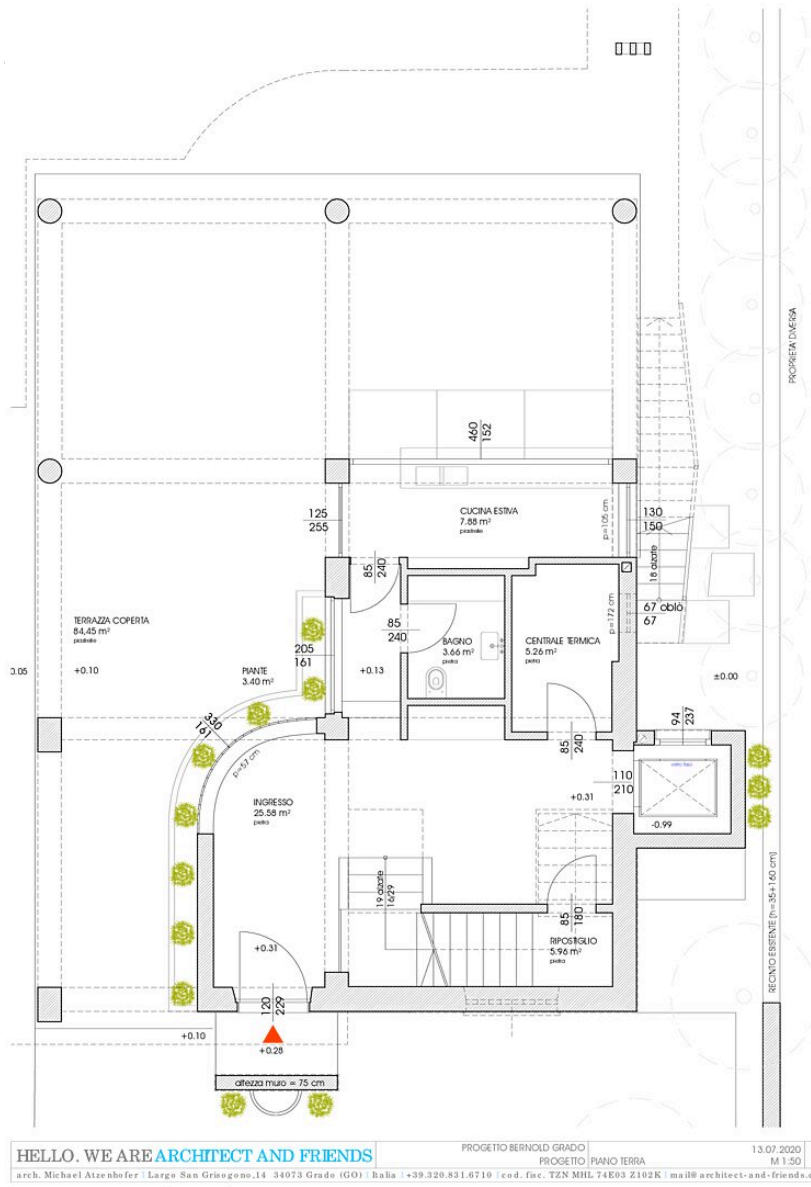
Grundriss EG
