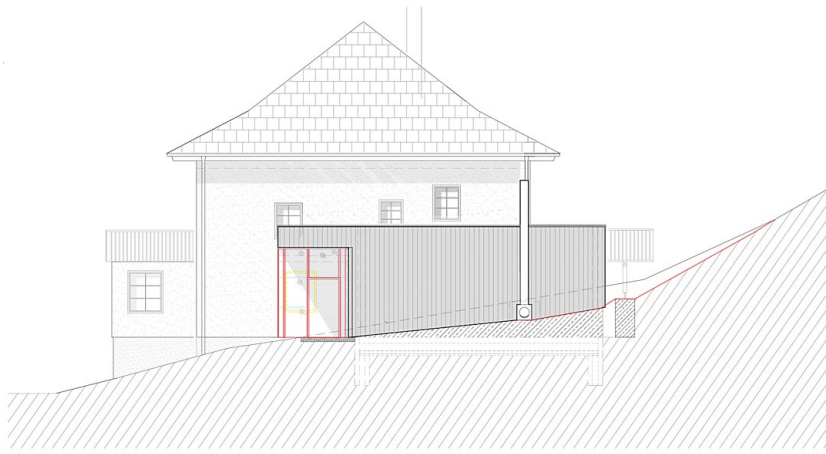
OSTANSICHT M 1:100
