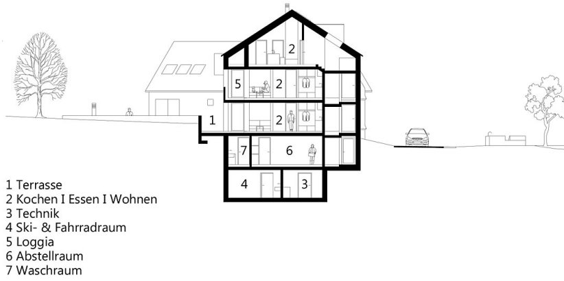
Querschnitt Haus B
