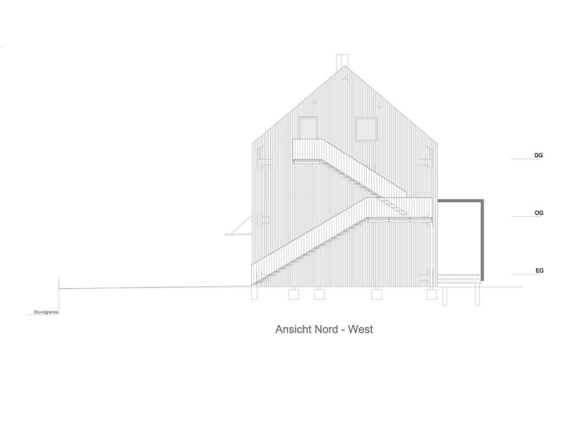
Ansicht Nord West
