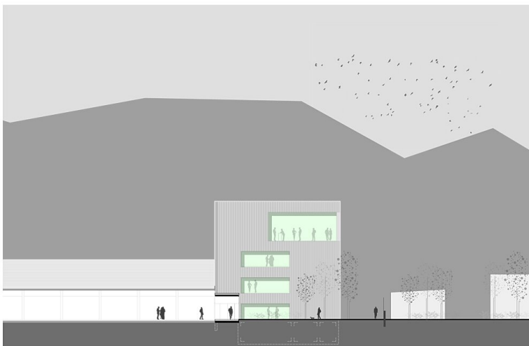
Ansicht Nord
