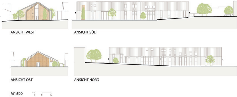
Ansichten
