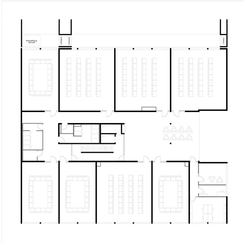
Grundriss Sockelgeschoß
