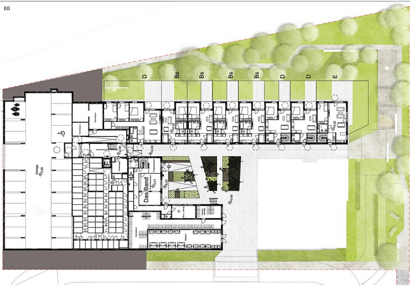
Grundriss EG
