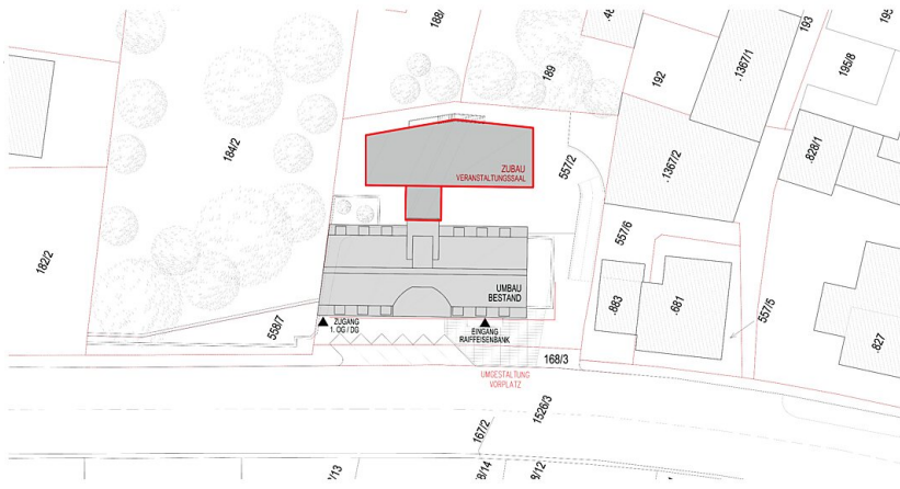
Lageplan
