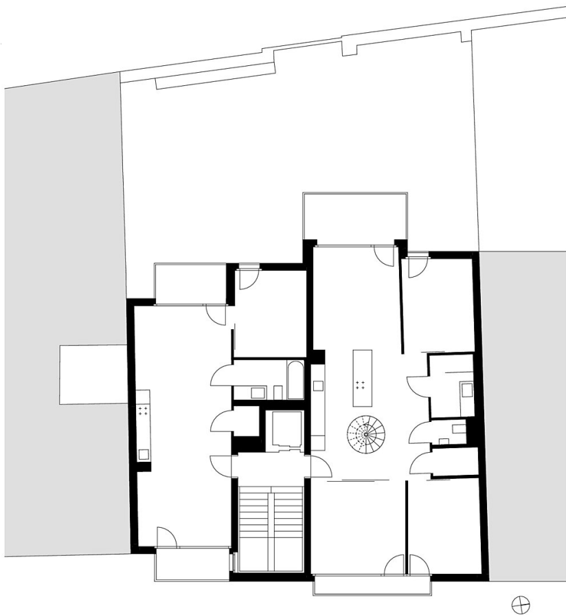
Grundriss OG2
