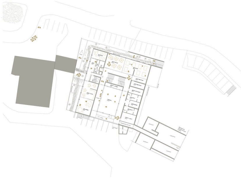
Grundriss UG
