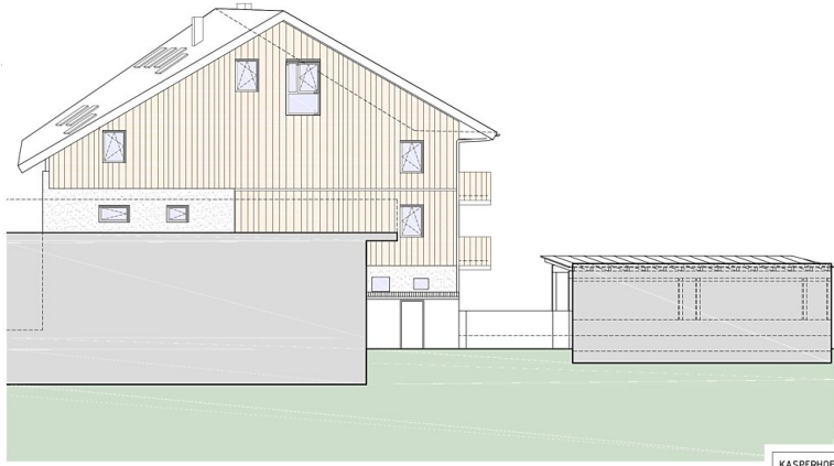
KASPERHOF 09/2018 ANSICHT WEST M. 1:100 architekturlokal
