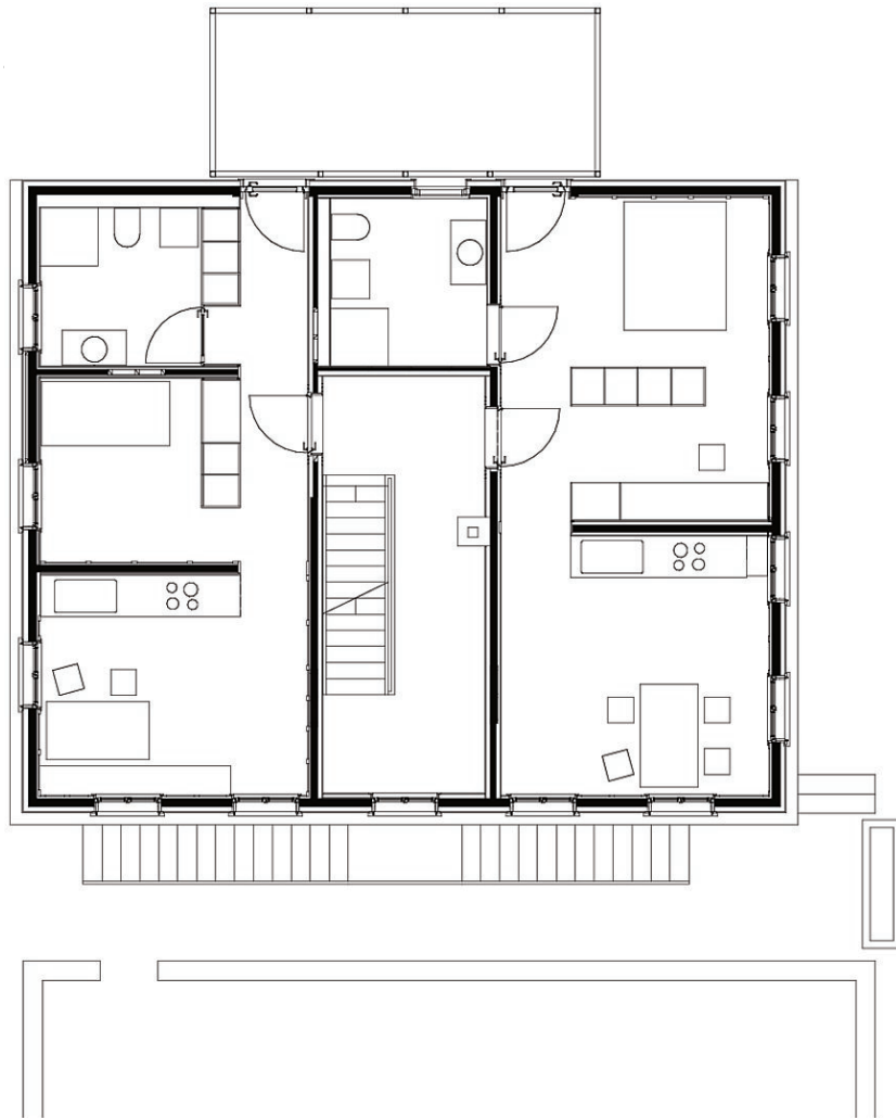
Grundriss OG
