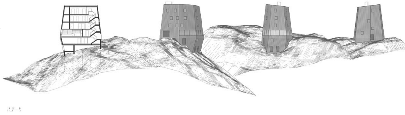
Ansichten & Schnitt
