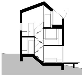
Schnitt 1 M 1:100
