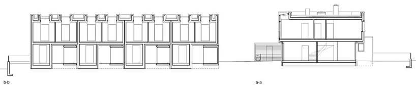
SCHNITTE 1:200
