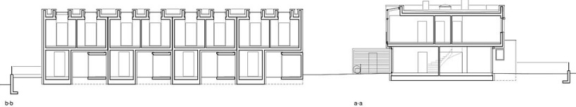
SCHNITTE 1:200
