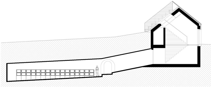
Grundriss, Schnitt
