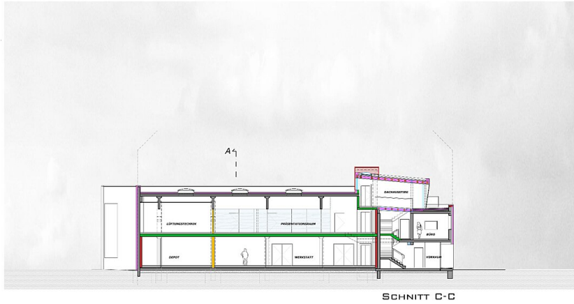
Schnitt CC
