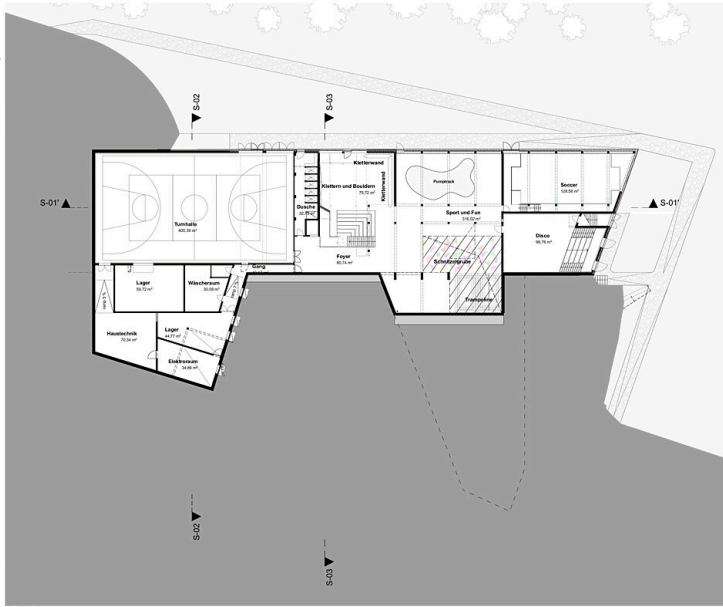
Jugendgästehaus Gerlosplatte -2. Untergeschoss M 1:200 Kochner - Kochner - Kochner ZT gmbH Praxiswegungasse 18, A-1020 Gatstorf
