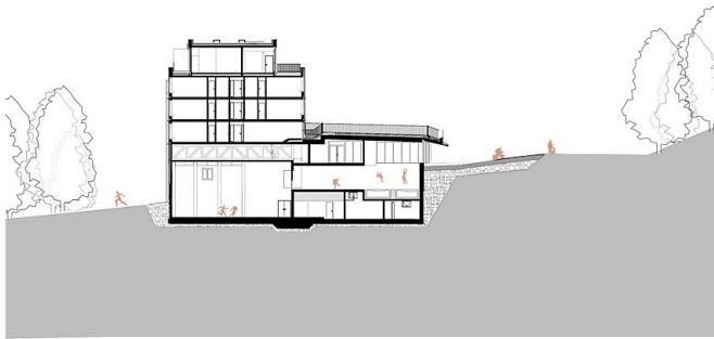
Jugendgastehaus Gerlosplatte Schnitt Turnhalle M 1:200 Kochner - Kochner - Kochner ZT gmbH Praxiswegungasse 18, A-1020 Gatstorf
