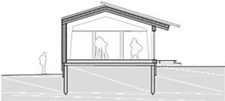
Schnitt BB'
