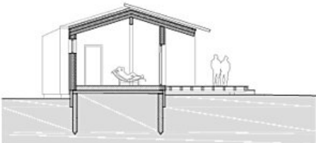
Schnitt AA'
