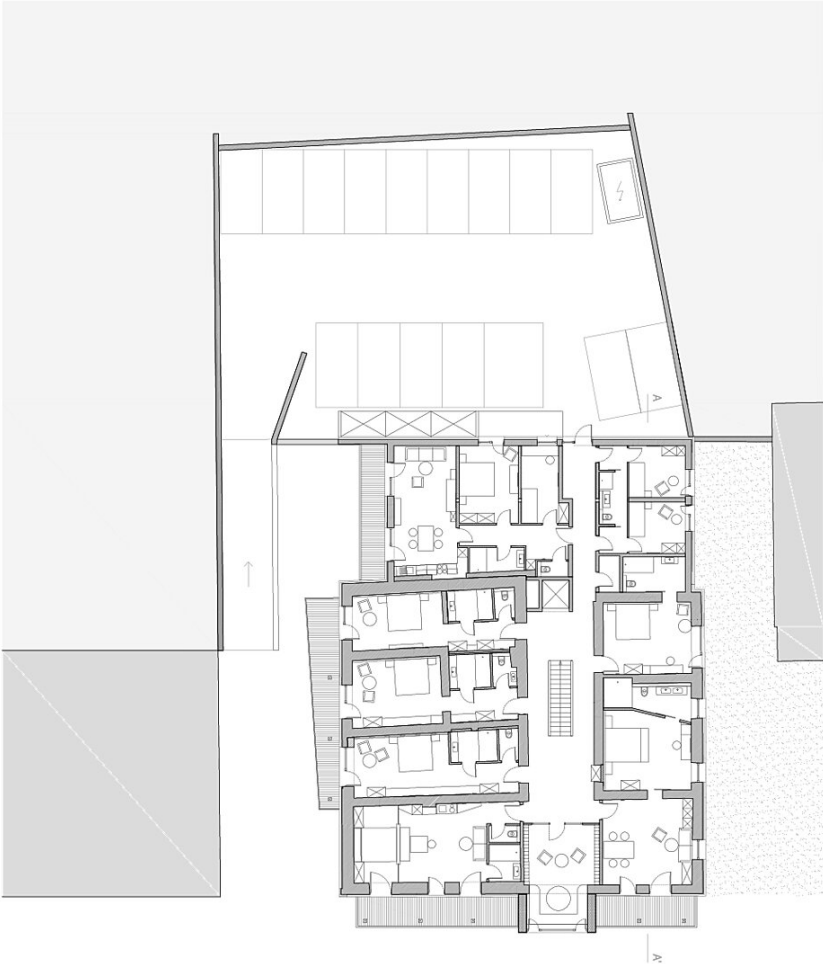
Grundriss OG1
