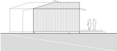
Nordansicht
