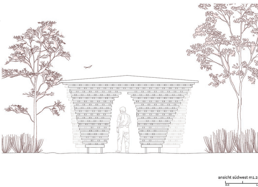
Ansicht
