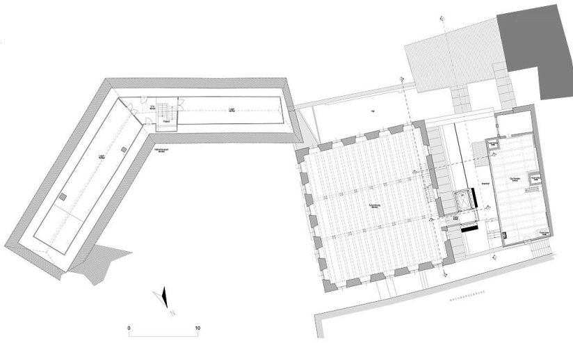
Grundriss OG2
