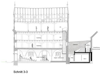
Schnitt 3-3
